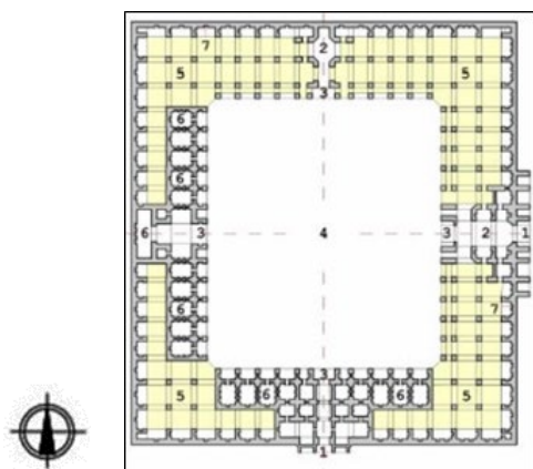
شکل ۱۵. نقشه برش‌های عمودی و پلان با مقیاس ۱:۲۰۰ کاروان سرای شاه‌عباسی لات (Zaraci, 2017)
