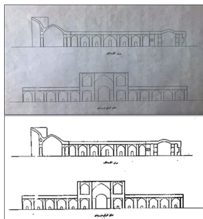
شکل ۱۵. نقشه برش‌های عمودی و پلان با مقیاس ۱:۲۰۰ کاروان سرای شاه‌عباسی لات (Zaraci, 2017)
