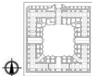
شکل ۶. برش‌های عمودی و پلان با مقیاس ۱:۳۵۰ کاروان‌سرای شاه‌عباسی کرج (Safa Mansouri, 2022)
