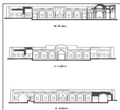
شکل ۱۳. نقشه برش‌های عمودی و پلان با مقیاس ۱:۳۰۰: کاروان‌سرای خزران
