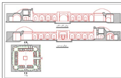
شکل ۹. نقشه برش‌های عمودی و پلان با مقیاس ۱:۵۰۰ کاروان‌سرای بنگی امام (Alborz, 2017)
